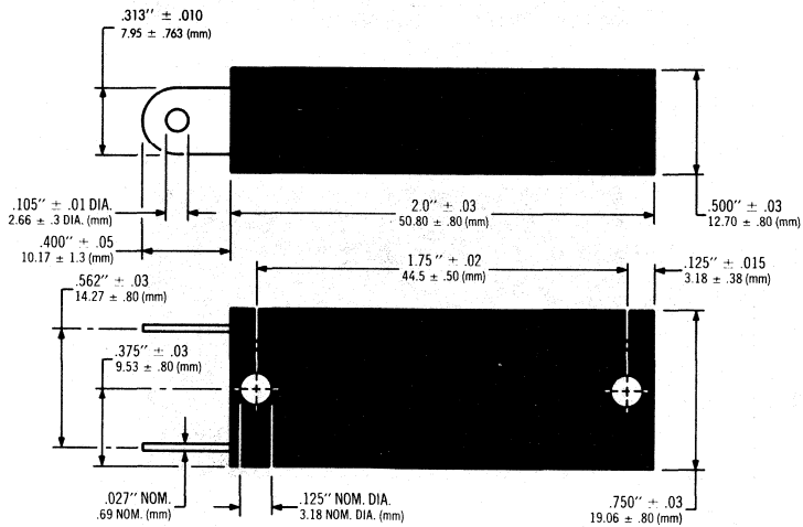
Case 2
