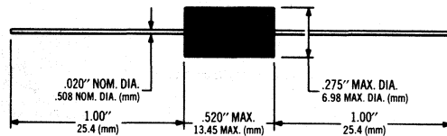
Case 9
