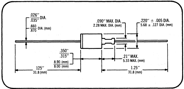
DO-13
