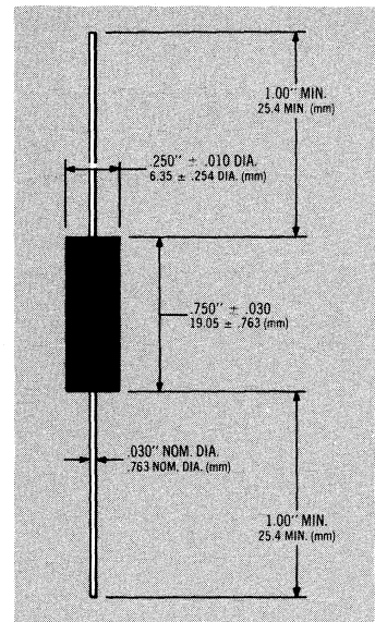
Case 19
