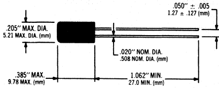
Case 5
