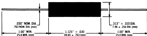
Case 20
