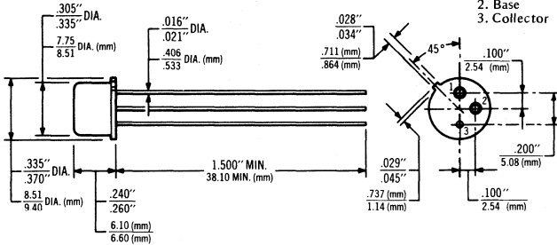
Case TO-5
