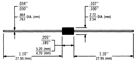
Case DO — 41
