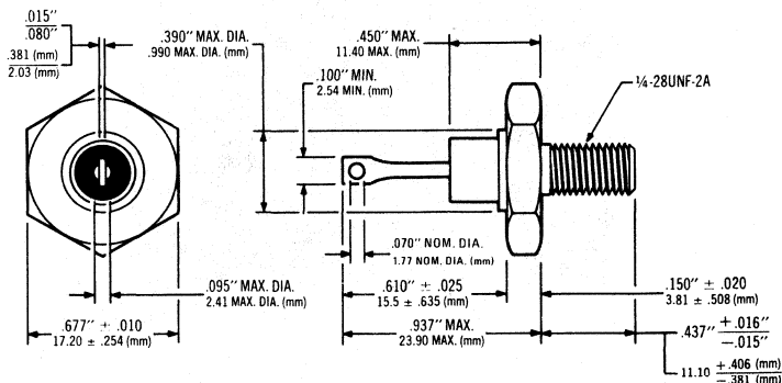
Case DO — 5, 1/4—28
