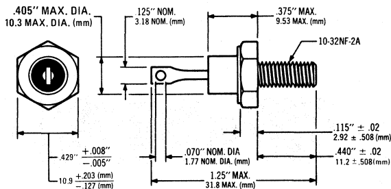
Case DO — 4, 10 — 32
