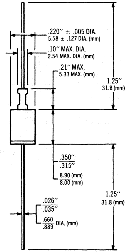
Case DO—13
