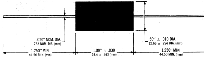
Case 16
