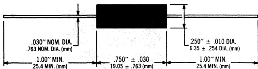
Case 19
