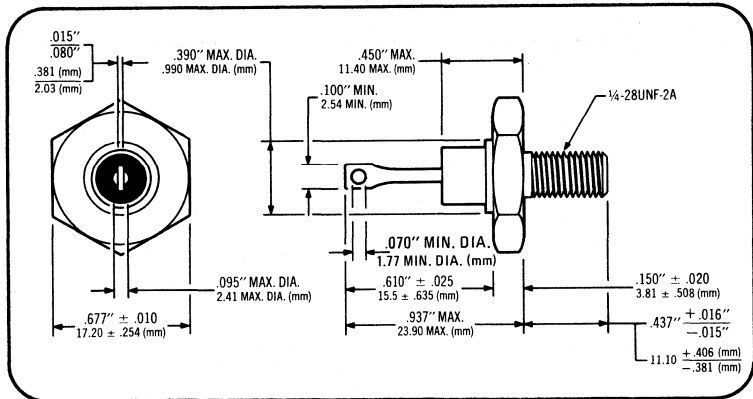
DO-5, 1/4-28
