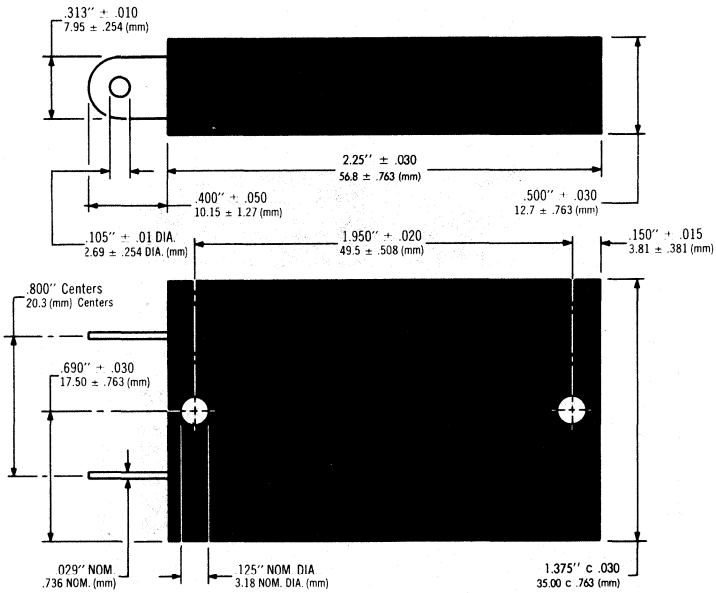
Case 4
