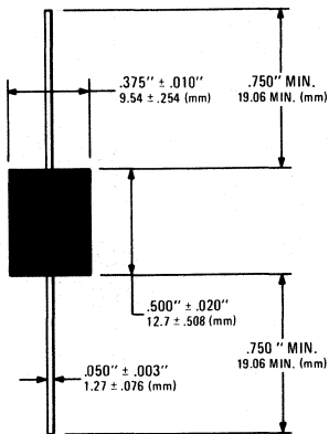
Case 23
